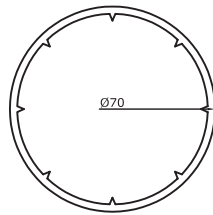
7021 Eksenel Dönüş Borusu Corner Pipe 0,850 kg/m
